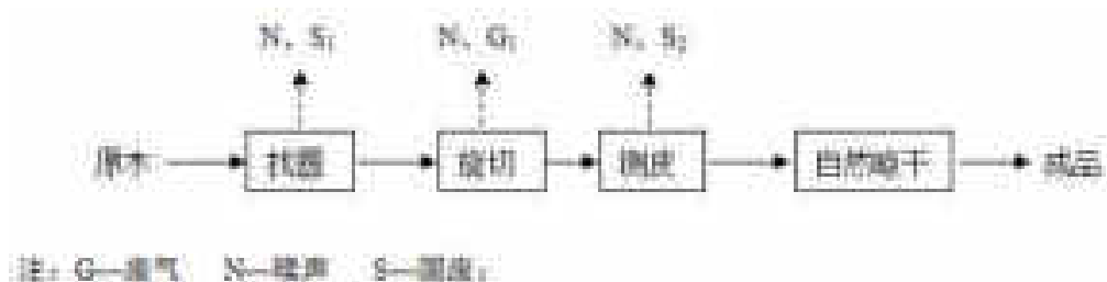
图 4-2 木皮生产工艺流程及产污环节图
