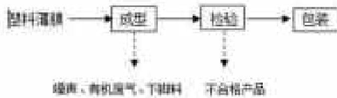
图 4-7 手套厂生产工艺流程及产污环节图
