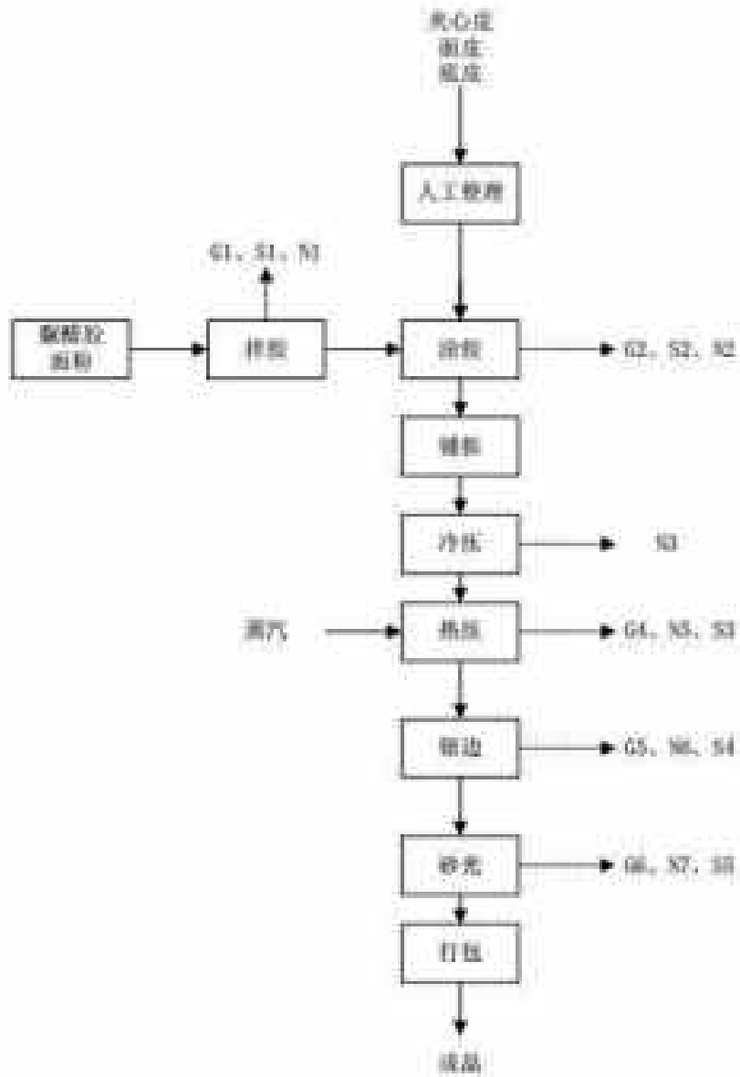
图 4-1 胶合板生产工艺流程及产污环节示意图
